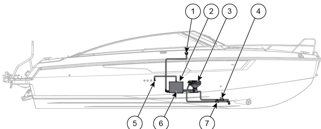
Figur 11.1 Yamarin 88 DC avloppssystem
