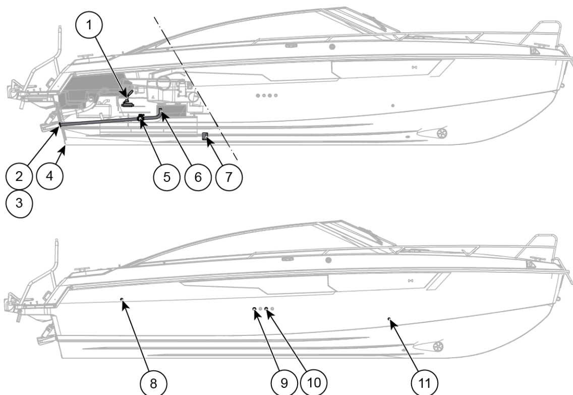
Figur 9.1 Yamarin 88 DC länspumpar och dränering
