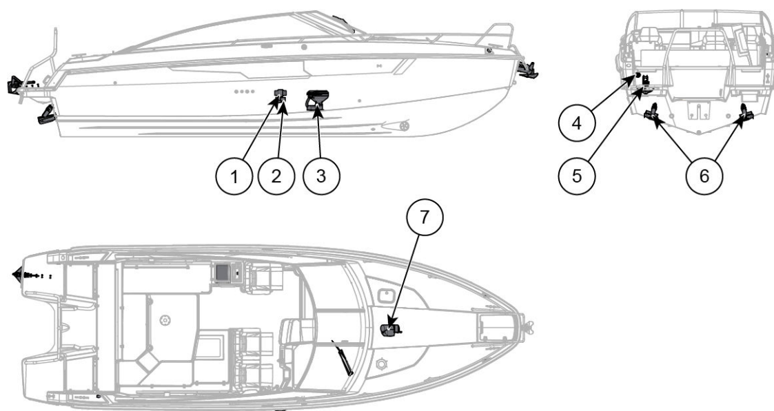
Figur 8.2 Yamarin 88 DC elektrisk utrustning
