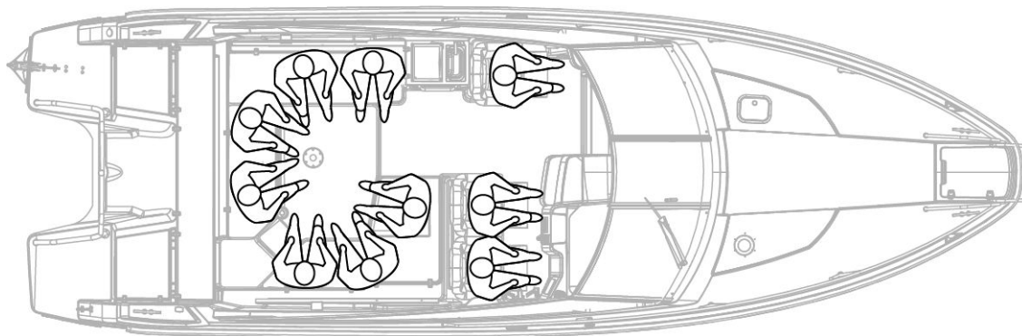
Figur 4.1 Yamarin 88 DC sittplatser för maximalt tio (10) passagerare
