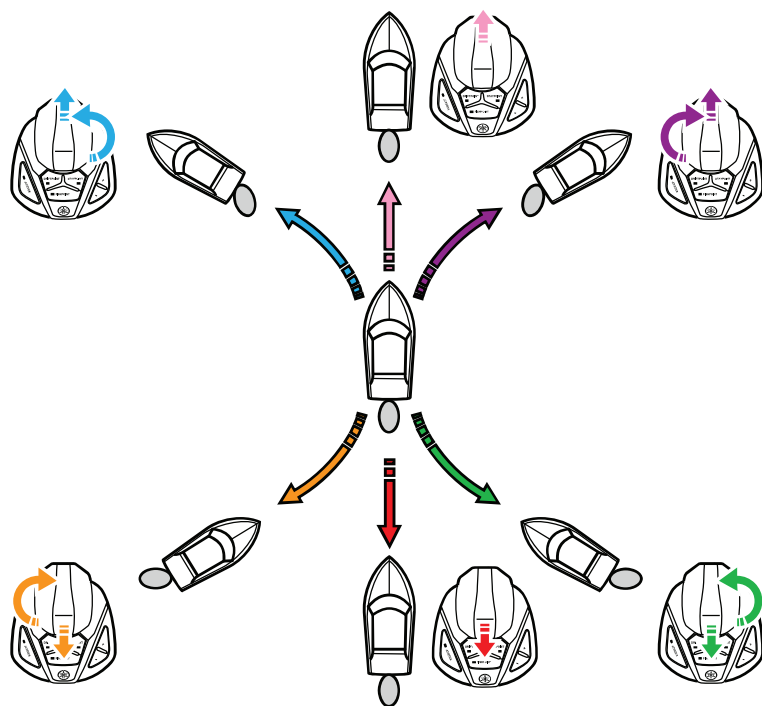
Figur 5.4 Drift av joystick med en enmotorig båt
