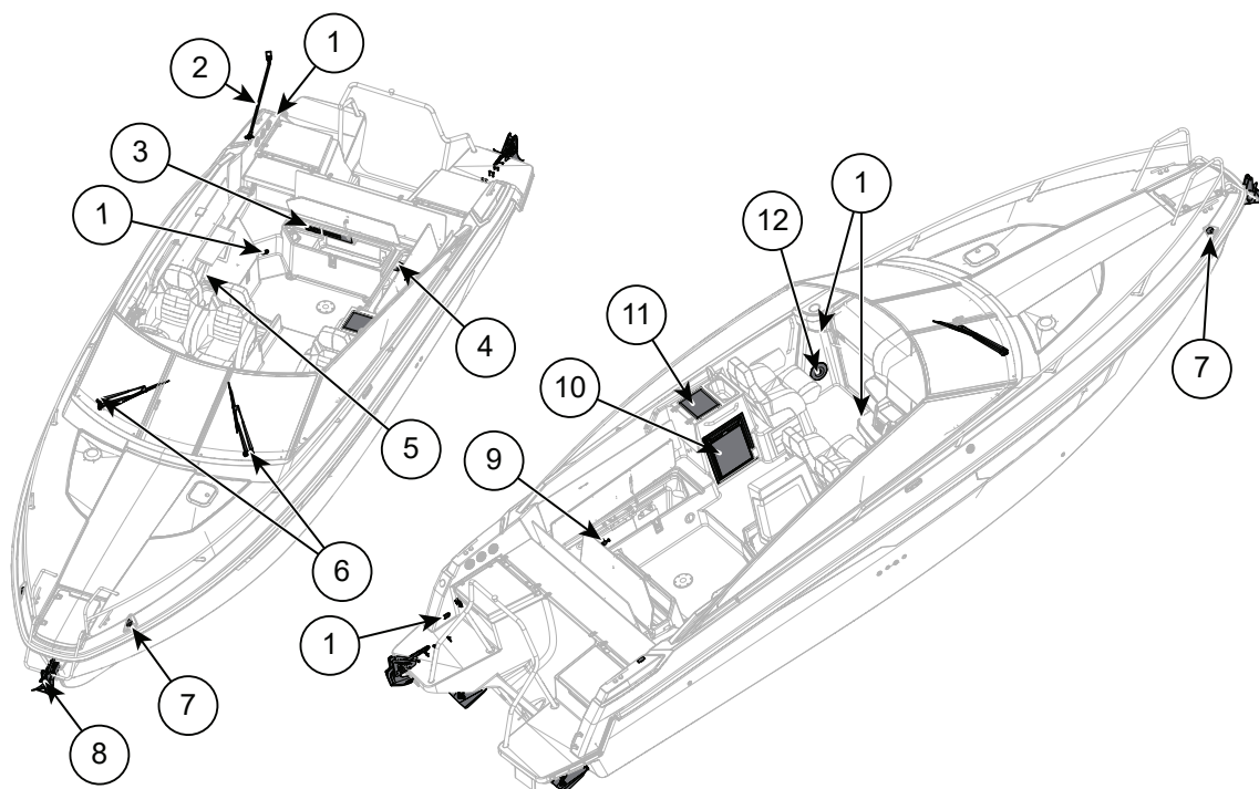
Figur 8.3 Yamarin 88 DC elektrisk utrustning
