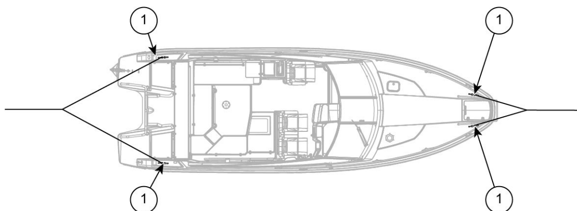
Figur 5.6 Yamarin 88 DC förtöjnings- och bogseringspunkter
