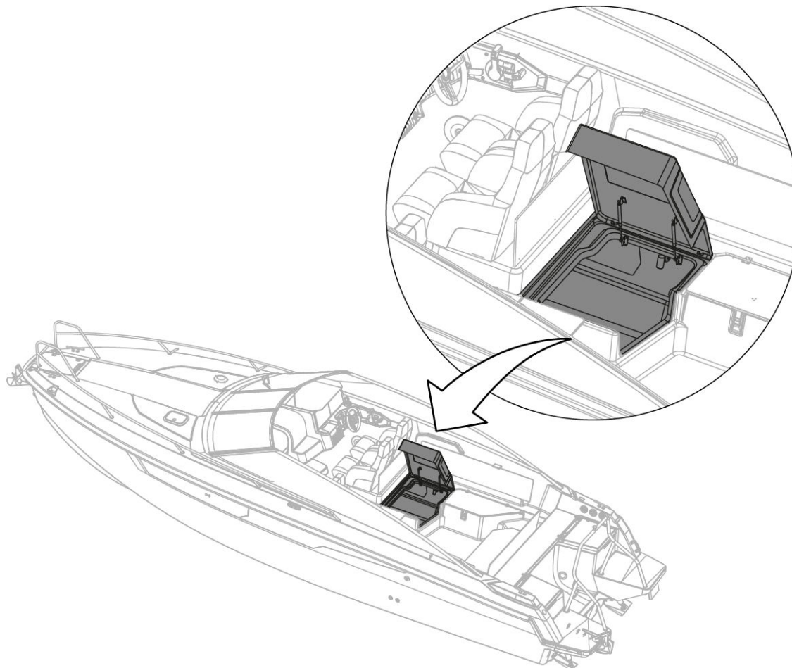
Figur 4.2 Åtkomstlucka till mittkabin
