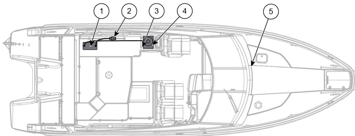
Figur 6.2 Yamarin 88 DC bränsle driven utrustning
