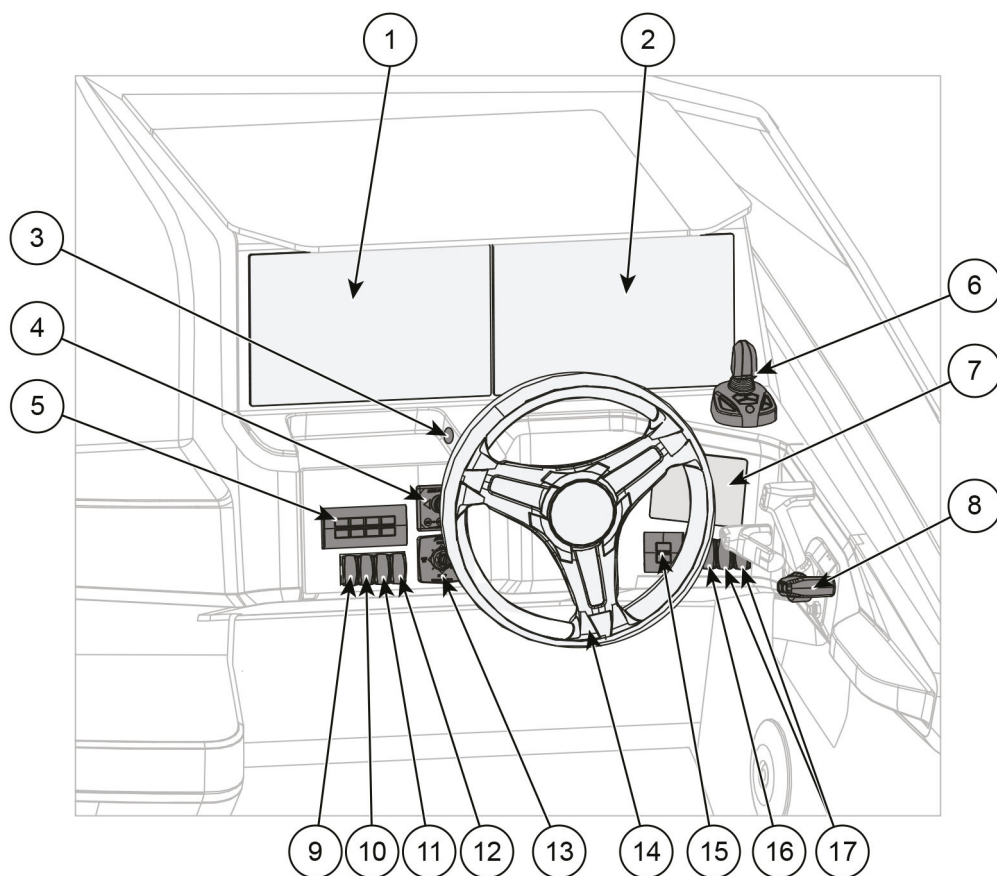
Figur 5.1 Yamarin 88 DC förarplatsens kontroller
